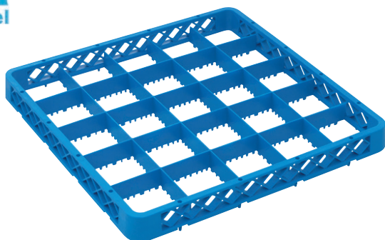
12633 RIALZO PER BASE 25 SCOMPARTI BLU cm 50x50 Dimensione scomparti cm 9x9 H 4,5
